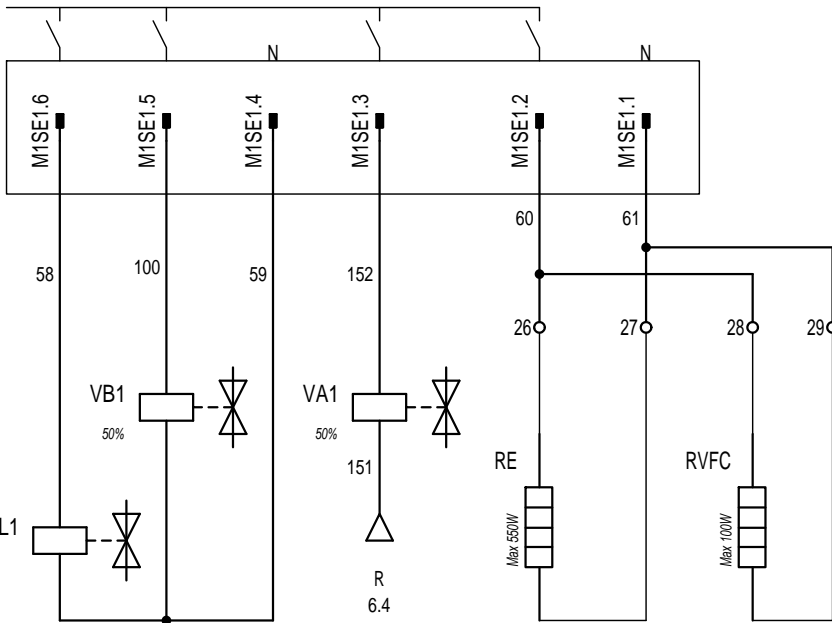
ANTIGELO EV. ANTIFREESE EV
